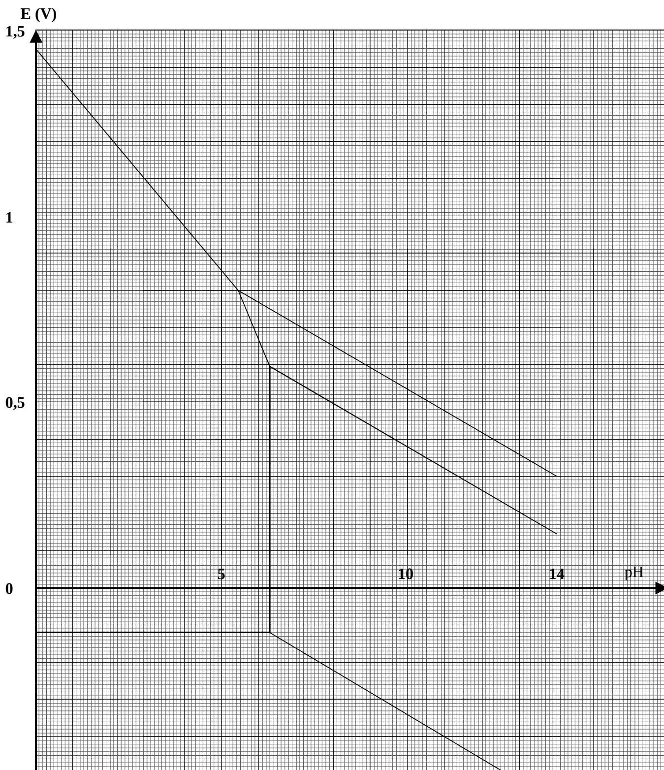
Figure 3 : Diagramme potentiel – pH simplifié de plomb
